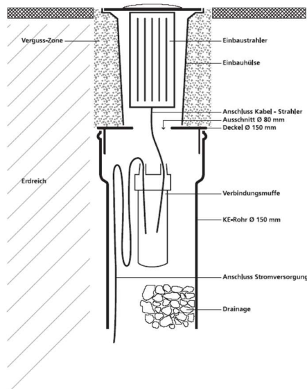
Kabelanschluss mit jederzeit wieder trennbarer Heitronic Verbindungsmuffe Art. 45605
