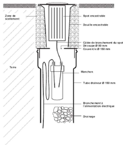
Branchement du câble avec le manchon dévissable Heitronic réf. art. 45605
